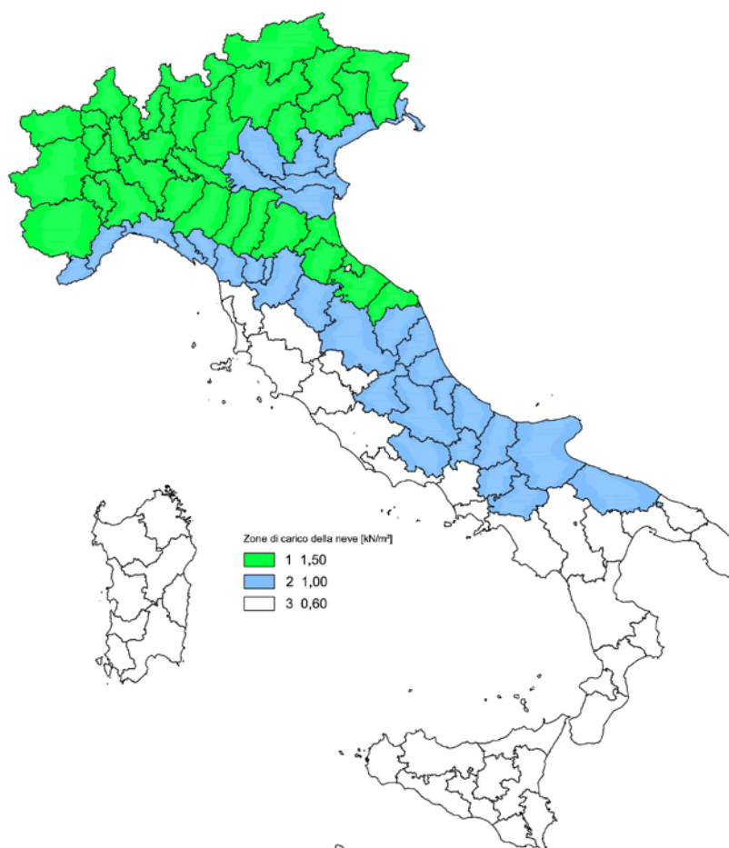
Fig. 3.4.1 – Zone di carico della neve
