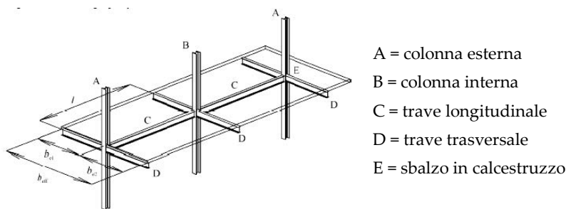
Fig. 7.6.2 - Definizione degli elementi in una struttura intelaiata
